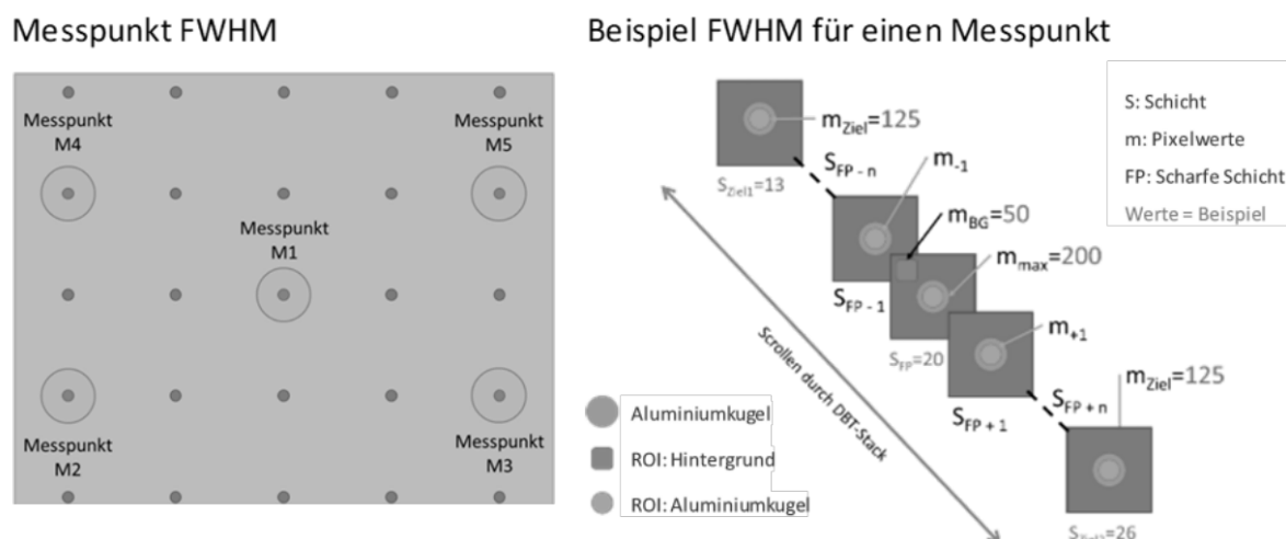
Abbildung E.2.10 – Messpunkte für die Bestimmung der FWHM-Werte
