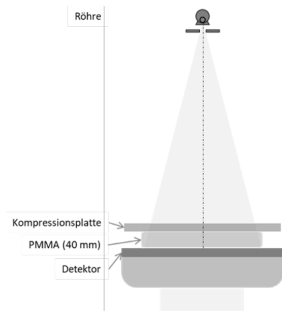
Abbildung E.2.11 – Messaufbau 2
