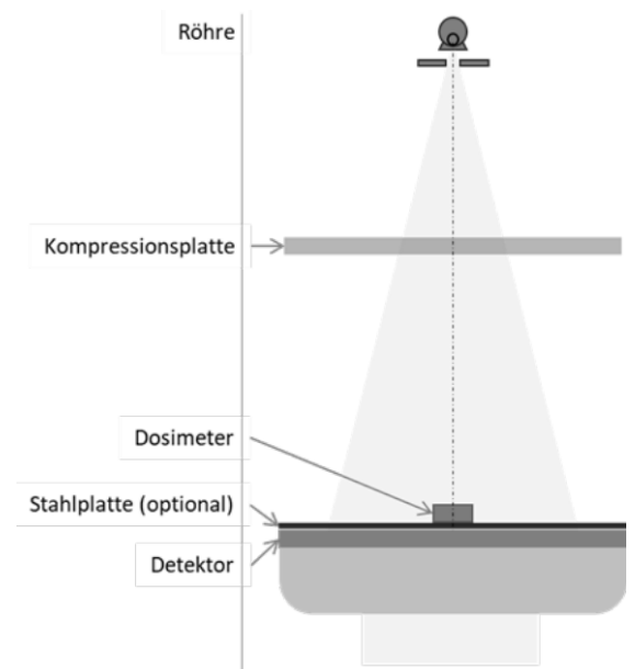
Abbildung E.2.2 – Messaufbau 1b
