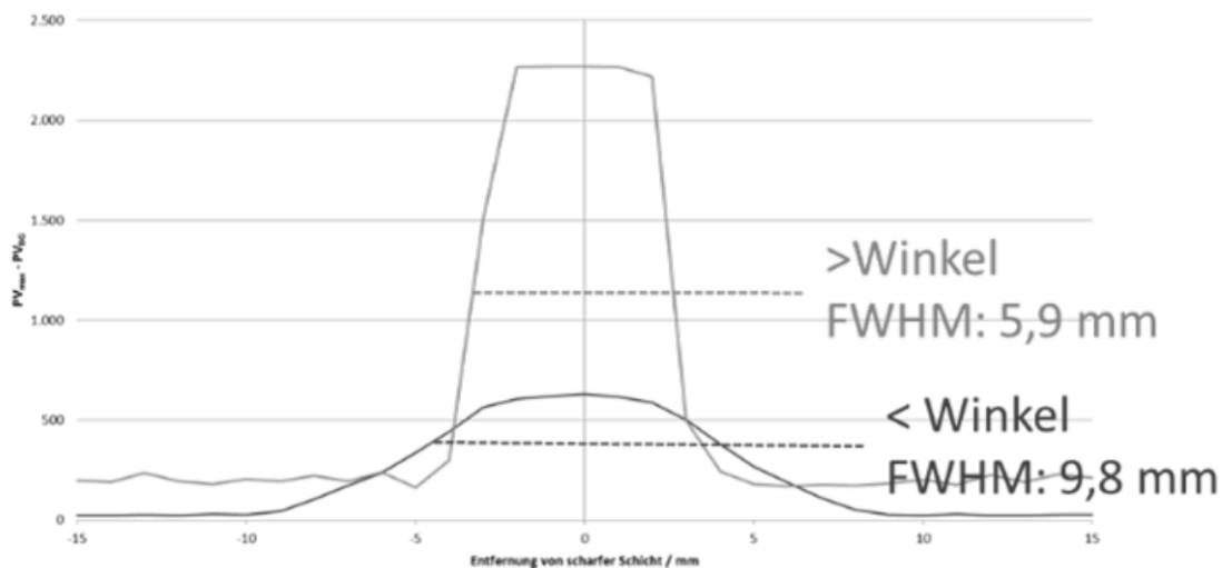
Abbildung E.7.1 – Beispiel FWHM und Kugelprofil
