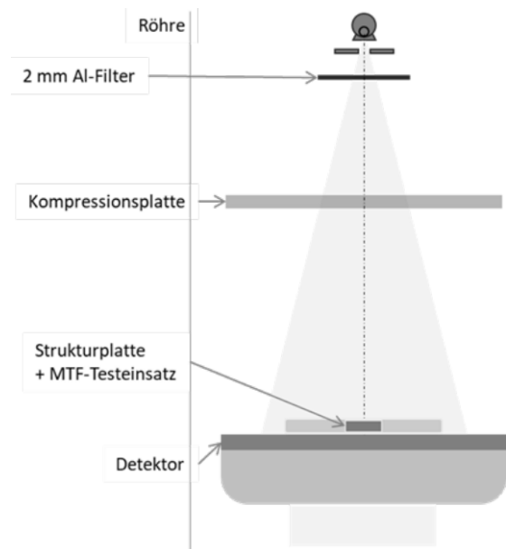
Abbildung E.4.2 – Messaufbau 8
