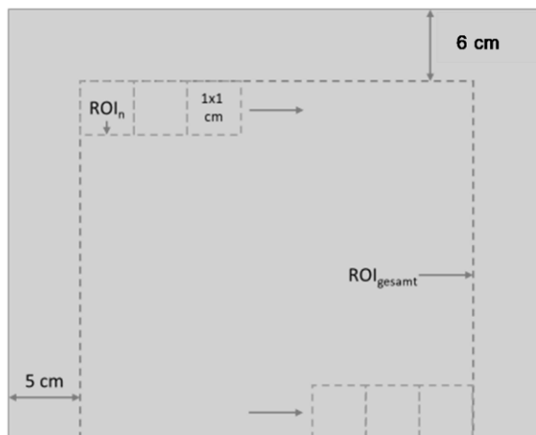
Abbildung E.2.12 – Schematische Darstellung der Auswertung der Homogenität
