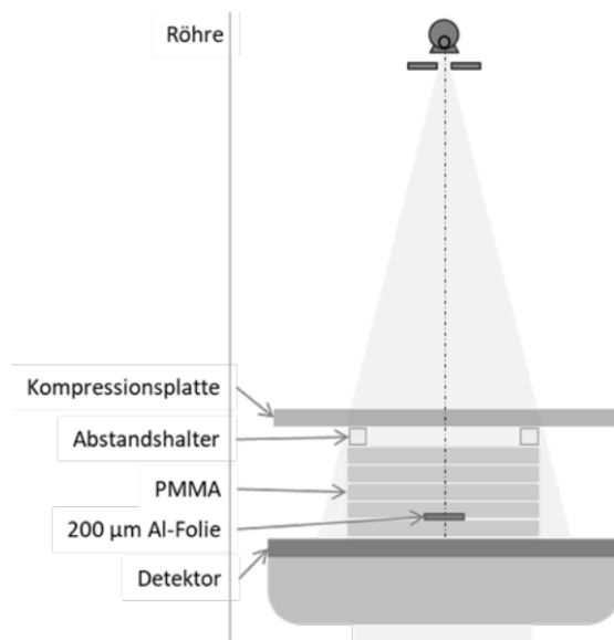
Abbildung E.2.3 – Messaufbau 3a
